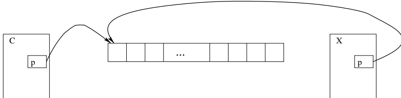
Рис. 10.1. Схема структуры данных после побитового копирования объекта
