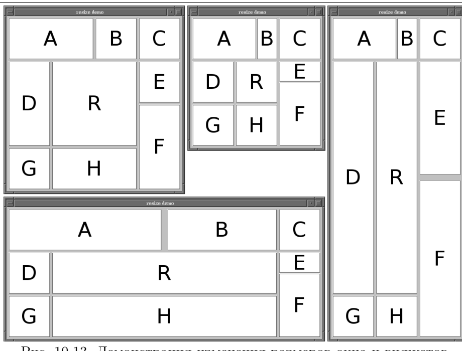
Рис. 10.13. Демонстрация изменения размеров окна и виджетов
