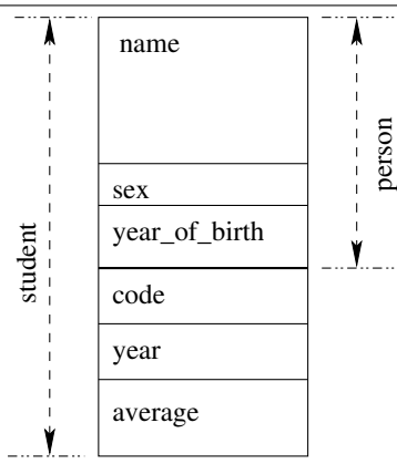
Рис. 10.3. Унаследованная структура данных
