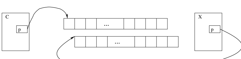
Рис. 10.2. Схема структуры данных после применения конструктора копирования
