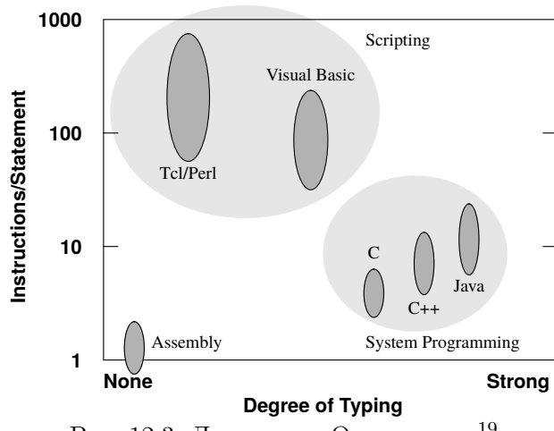
Рис. 12.3. Дихотомия Оустерхаута 19
