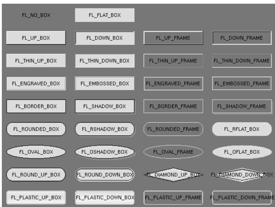
Рис. 10.9. Стили обрамления виджетов FLTK 34
